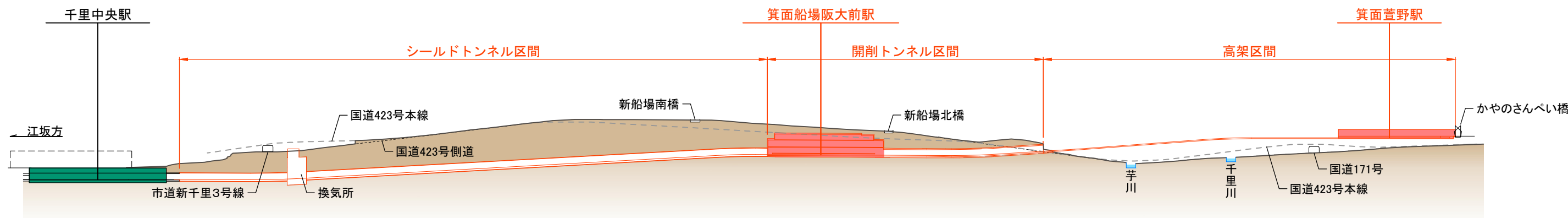
縦断面図
